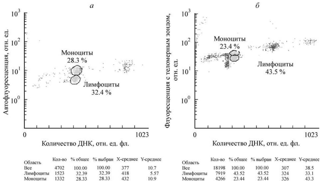
Рис. 2. Стандартная картина распределения клеточных событий по количеству ДНК (FL3, PI).
